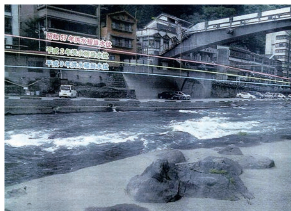
杖立川の洪水相当水位
